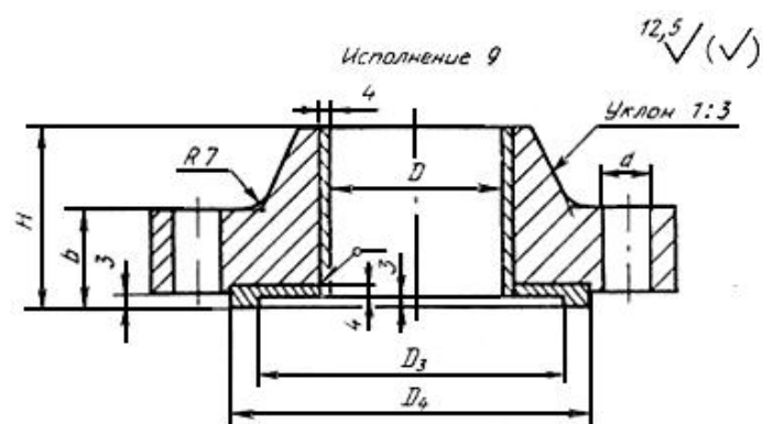
Черт.5 Исполнение 9 и 10
